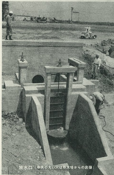
ダムの下流側法尻に設けられた導水路(手前は放水口)
