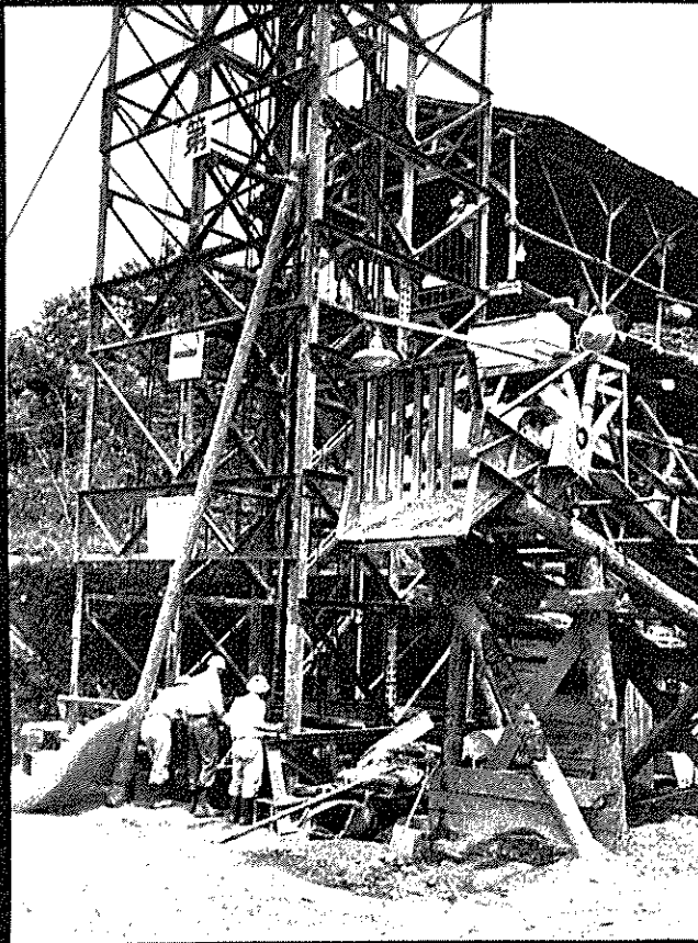
第1横坑入口、竖坑なので人も材料もエレベーターで昇降する
