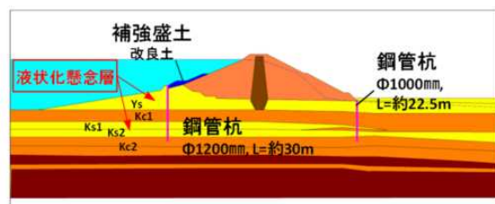
堤体補強工法
