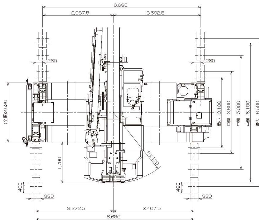
ラフタクレーン寸法(例)
