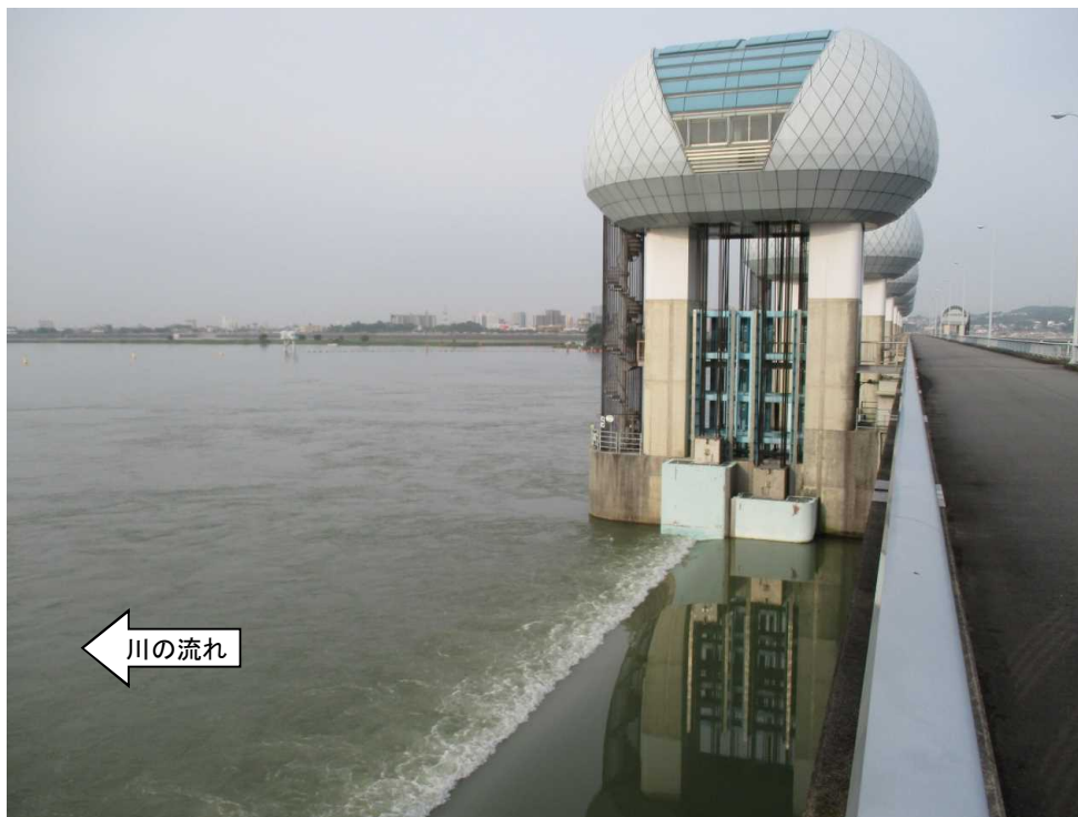
ゲート全開操作終了後の長良川河口堰（オーバーフロー操作に切り替え） 7月5日 6時撮影
