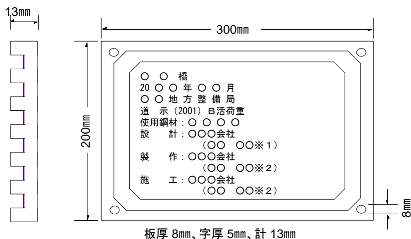
図3-2-2 銘板の寸法及び記載事項
