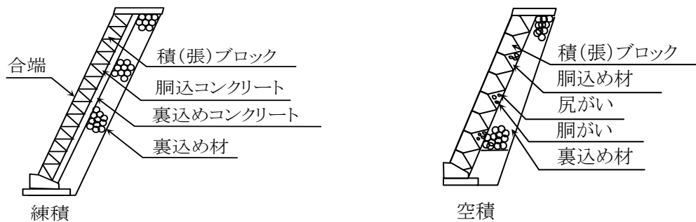
図3-2-5 コンクリートブロック工
