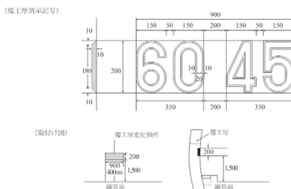
図10-6-1 覆工厚変化箇所の刻示標準図
