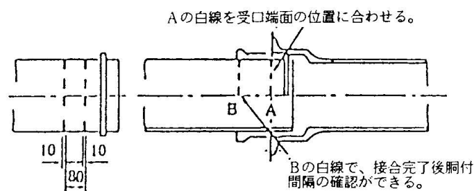
図11－3－1 受口・挿口の挿入完了位置 単位：mm
