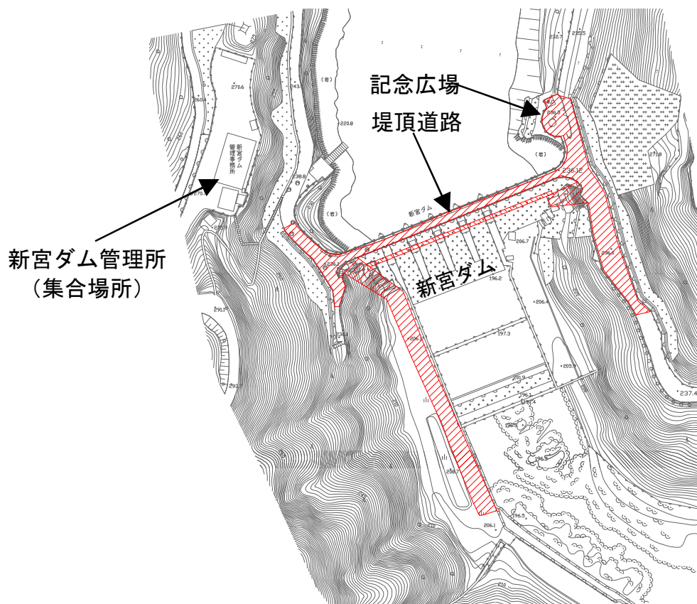
新宮ダム一般利用施設安全点検平面図
