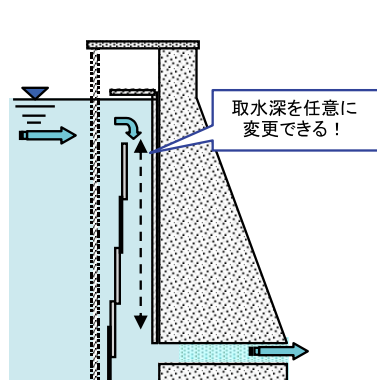
選択取水設備（イメージ図）
