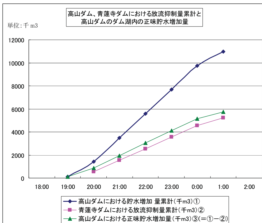
図ー２ 高山ダム、青蓮寺ダムにおける放流抑制量累計と 高山ダムのダム湖内の正味貯水増加量
