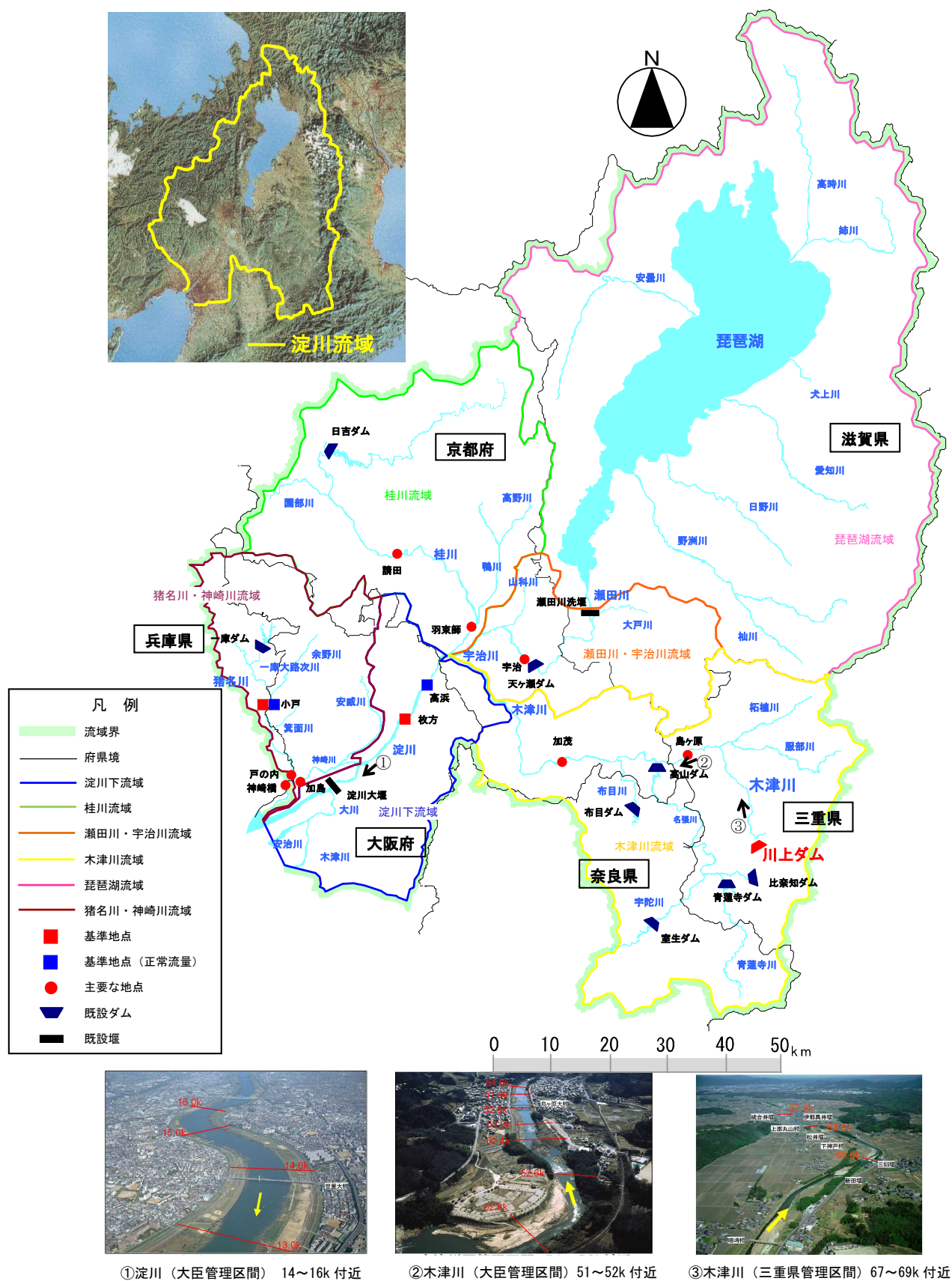
図 2.1-1 淀川流域図
