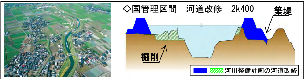
国管理区間河道掘削、築堤イメージ
