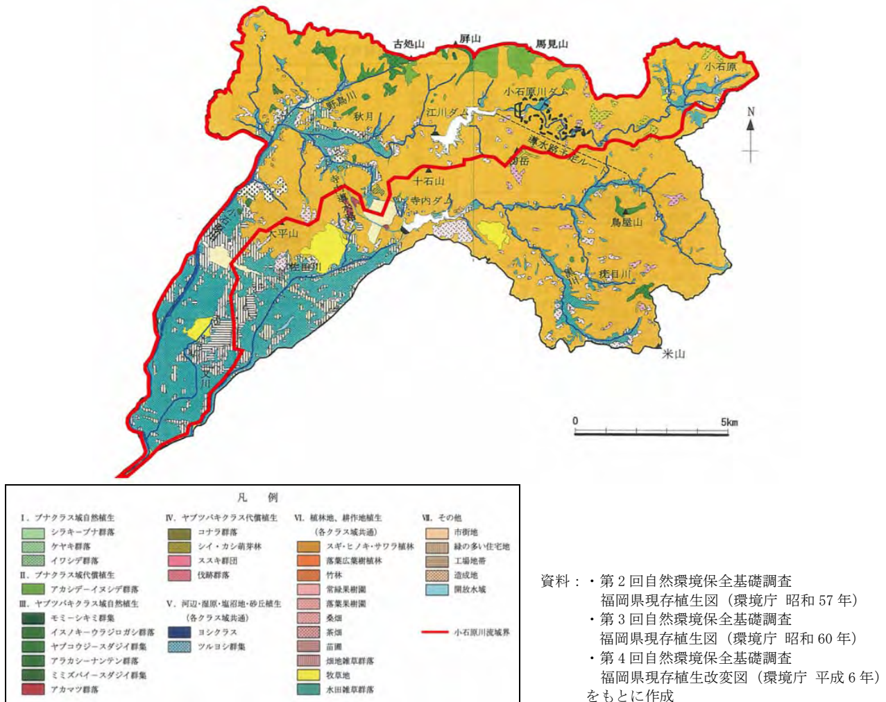
図 2.1-23 小石原川流域の植生図
