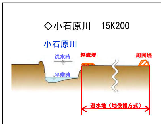
遊水地（地役権方式）イメージ
