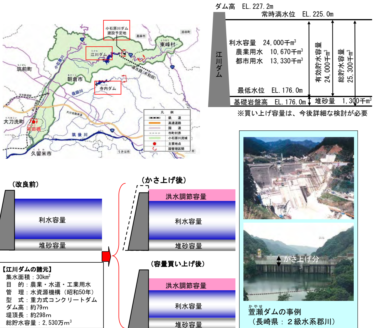
図 4.2-2 江川ダムの有効活用案のイメージ図
