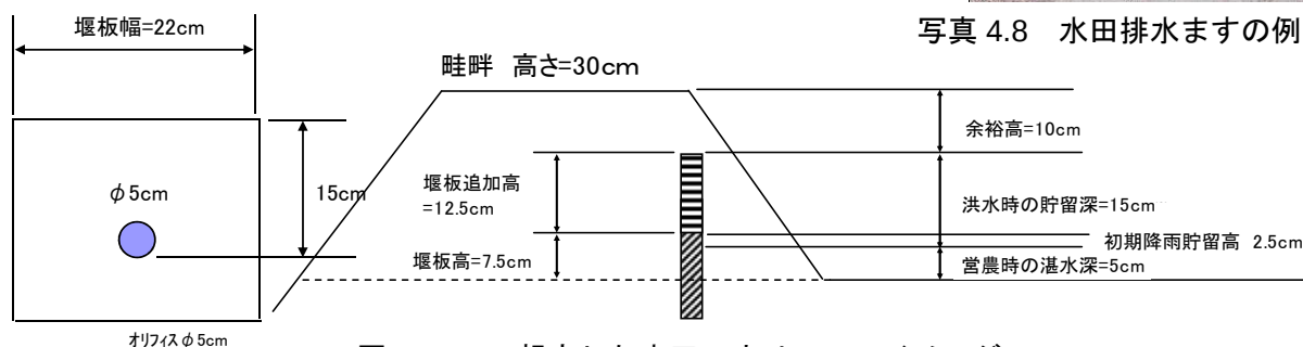
図 4.3.31 想定した水田のオリフィスイメージ
