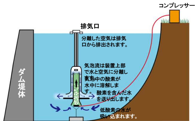
深層曝気設備の仕組み(イメージ図)※
