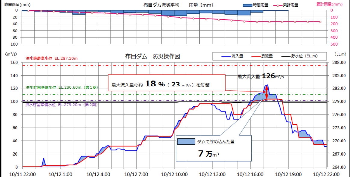
布目ダムの防災操作図
