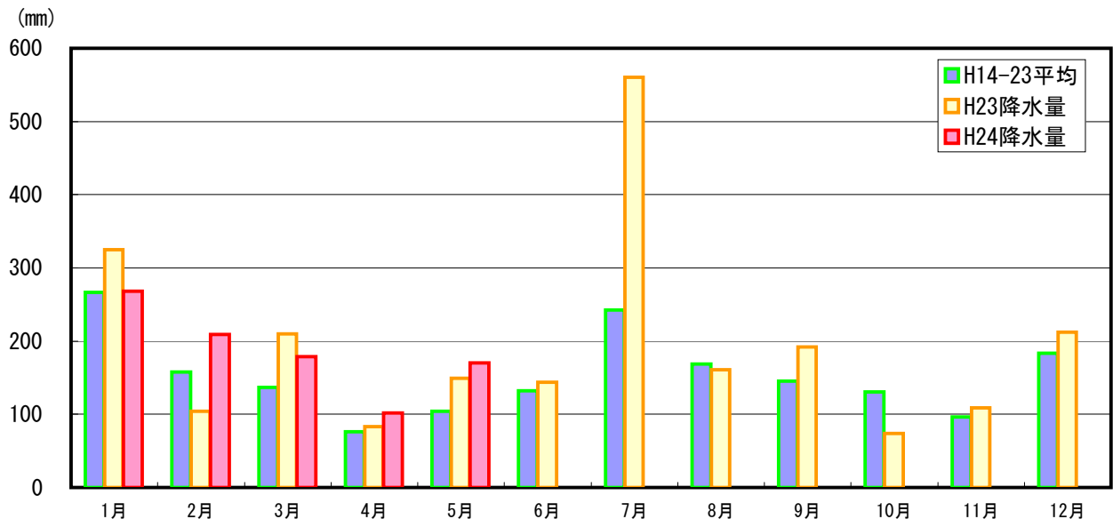
矢木沢ダム地点における降水量
