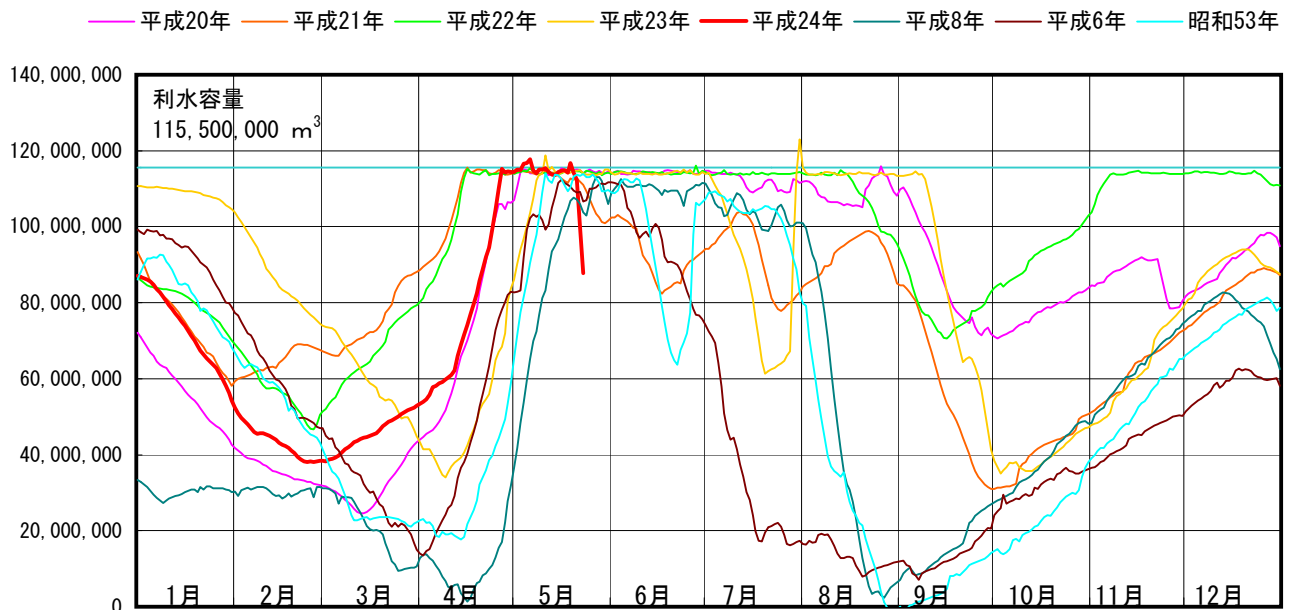
利水容量 (m 3 ) 矢木沢ダム利水容量曲線
