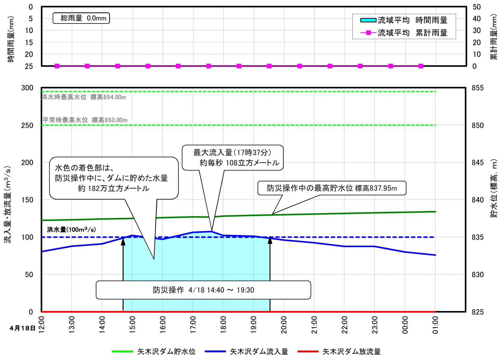
■ 矢木沢ダムの防災操作の状況図
