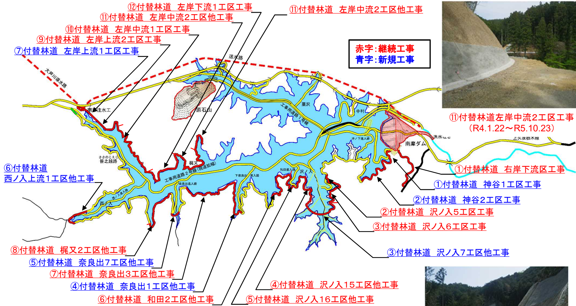
南摩ダム貯水池平面図
