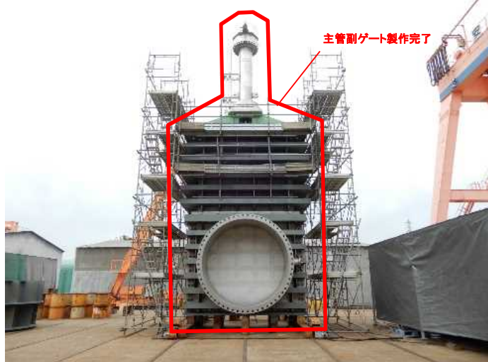
①主管副ゲート製作 施工状況(令和5年4月)
