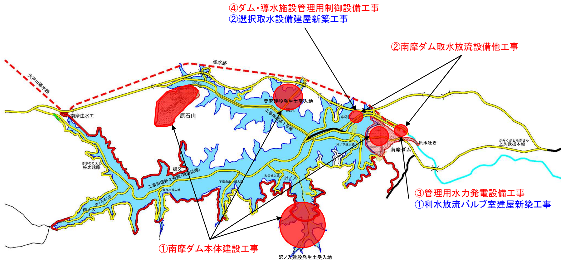
南摩ダム貯水池平面図
