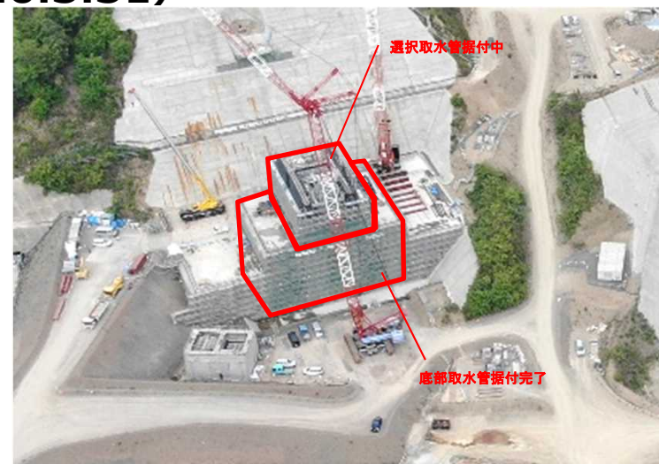
②取水管据付 施工状況(令和5年4月)
