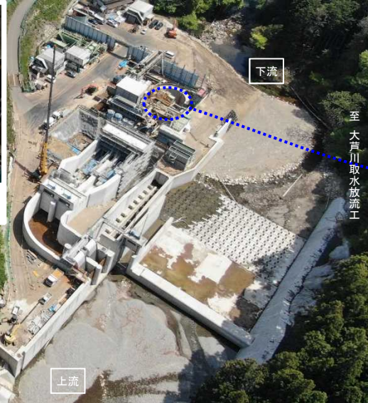
黒川取水放流工 施工状況(令和5年4月)
