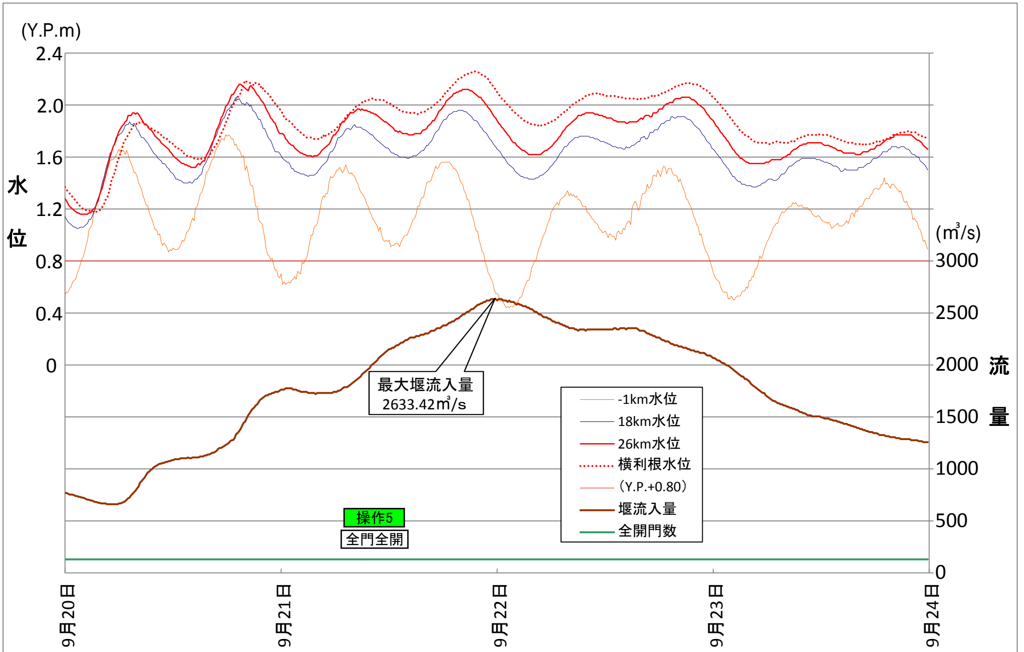
河口堰操作状況、堰上下流水位及び堰流入量
