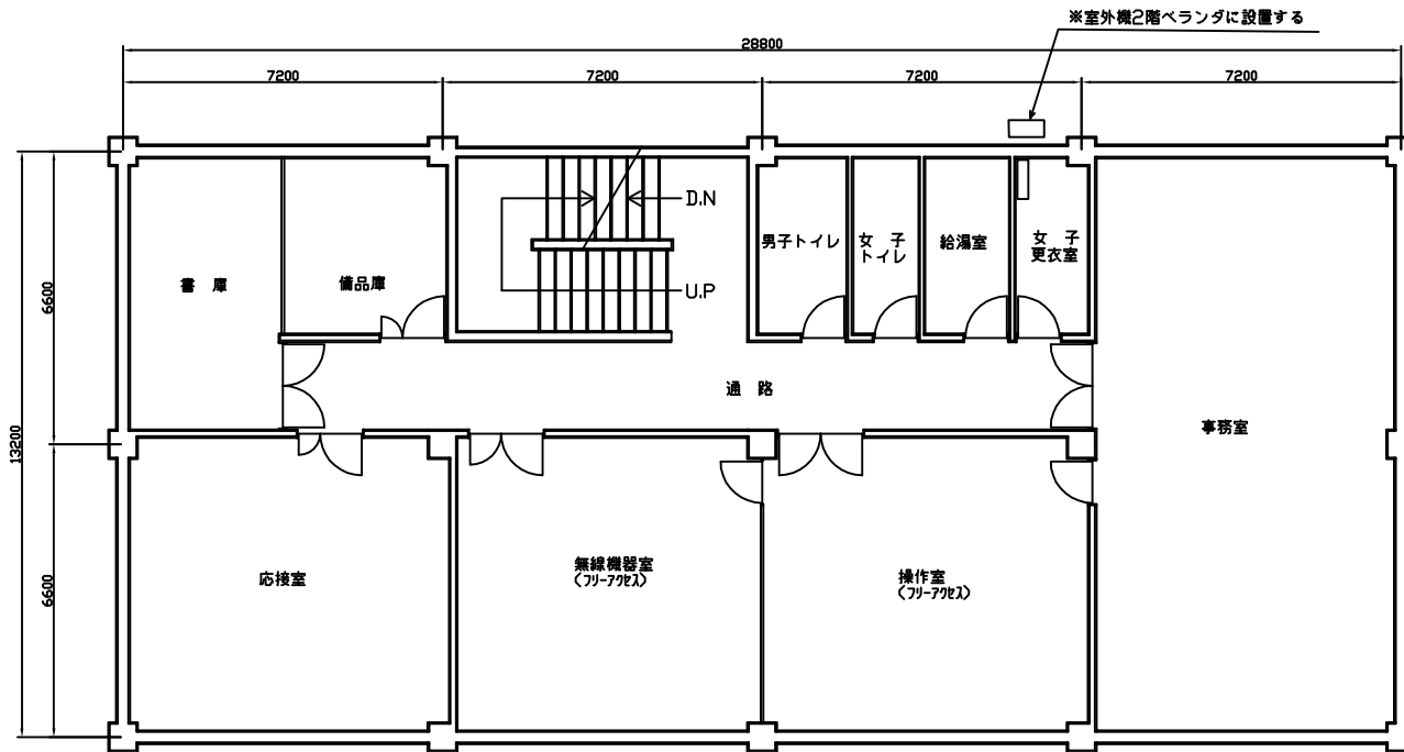
美濃加茂管理所2階平面図
