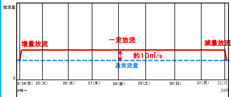
西平ダムの放流イメージ
