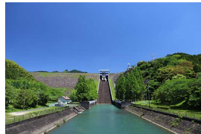
下流側からのゲート方向の状況
