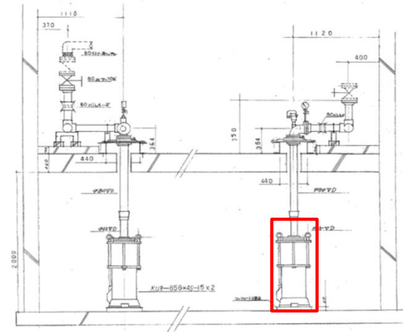
山見揚水施設 吸水槽断面図
