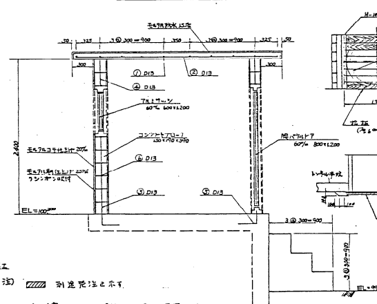
ポンプ室側面図 S=1/50
