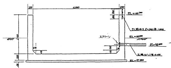
B-B断面図 S=1/50
