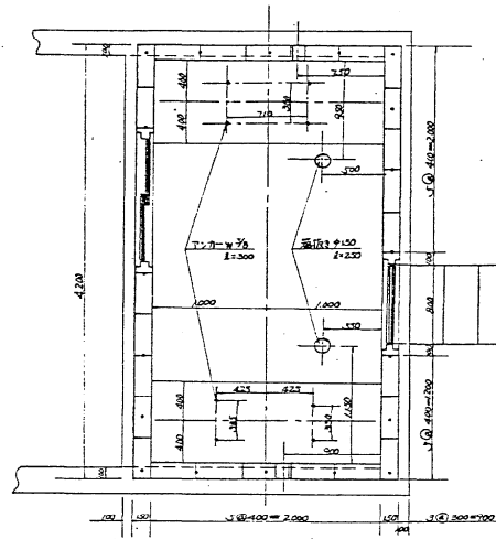
ポンプ室平面図 S=1/50
