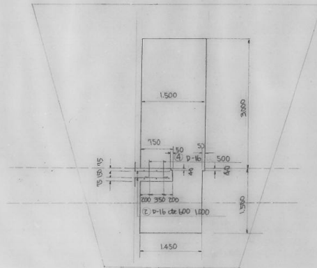
正面図 1/40
