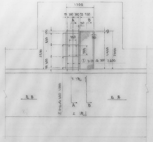
平面図 1/40
