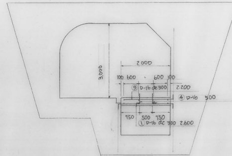
A-A断面 1/50
