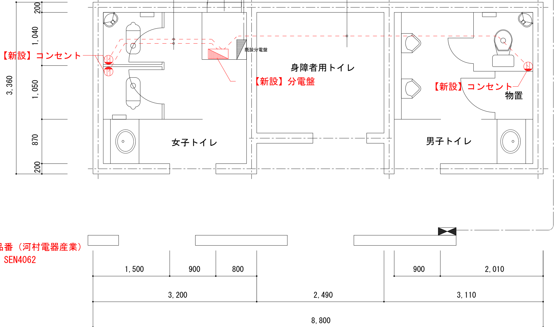
しもうけ館屋外トイレ電気設備改修平面図
