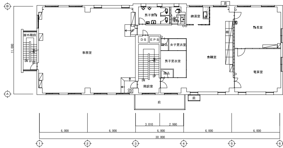
2階平面図
