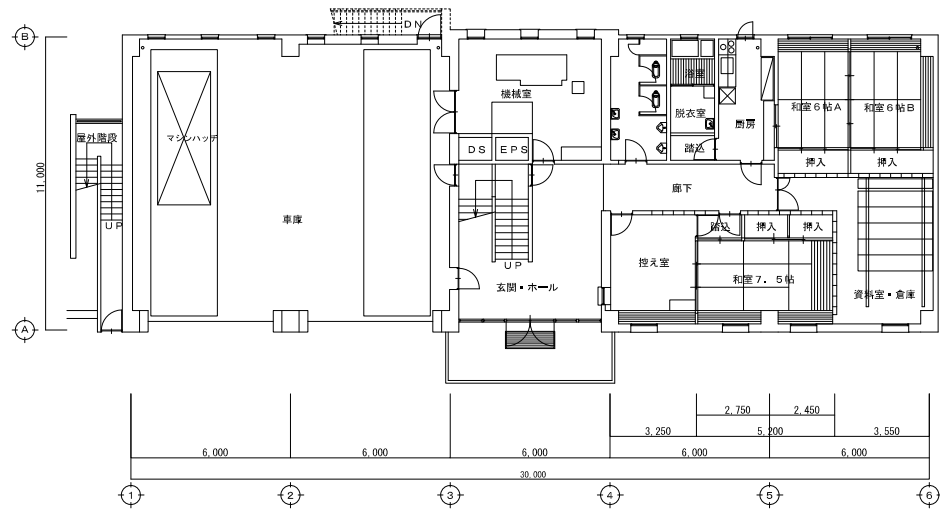
1階平面図
