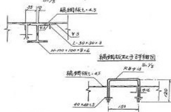
詳細図
