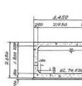
断面 E-E
