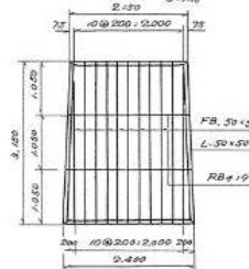
スクリーン戸当り詳細図
