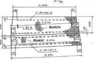
鋼網板詳細図
