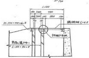
鋼網板取付部詳細図
