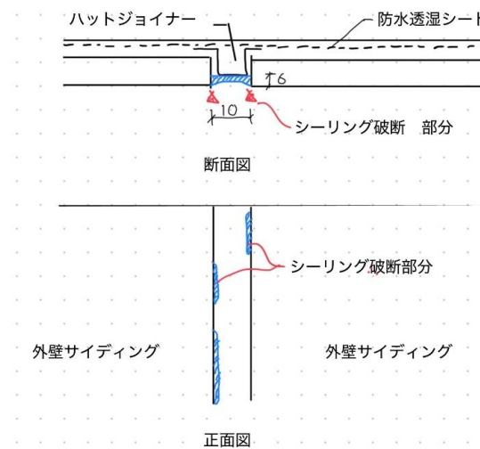
破断部拡大(1)
