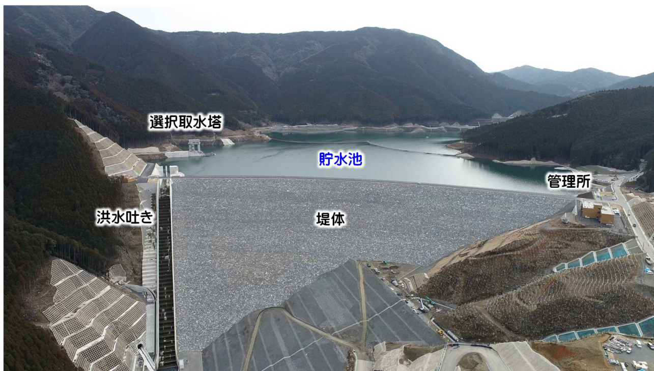
ダム堤体
