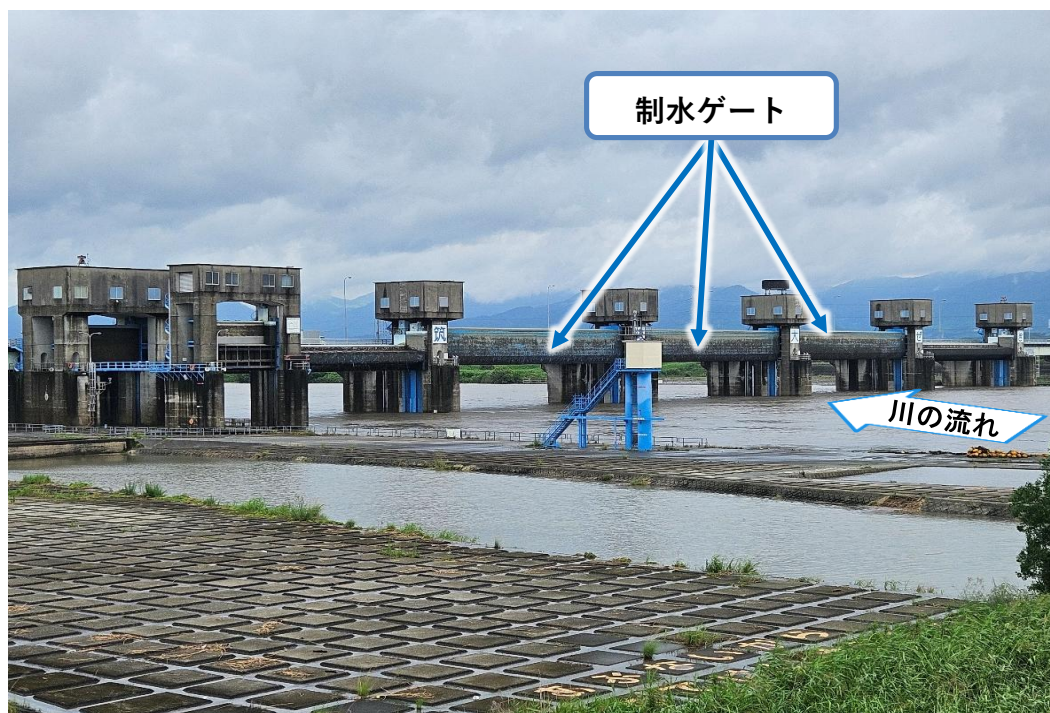
ゲート全開操作開始後の筑後大堰 (左岸上流側から筑後大堰を望む)
