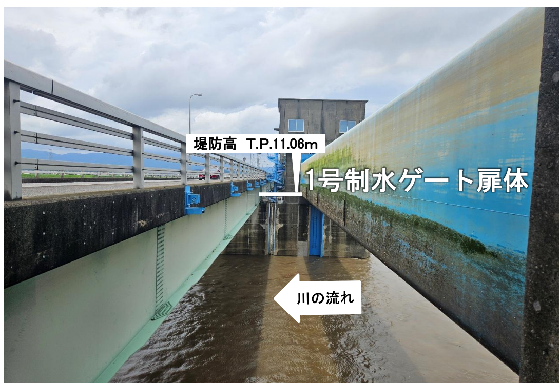
ゲート全開操作開始後の筑後大堰 (1号制水ゲートを左岸から右岸方向に望む)
