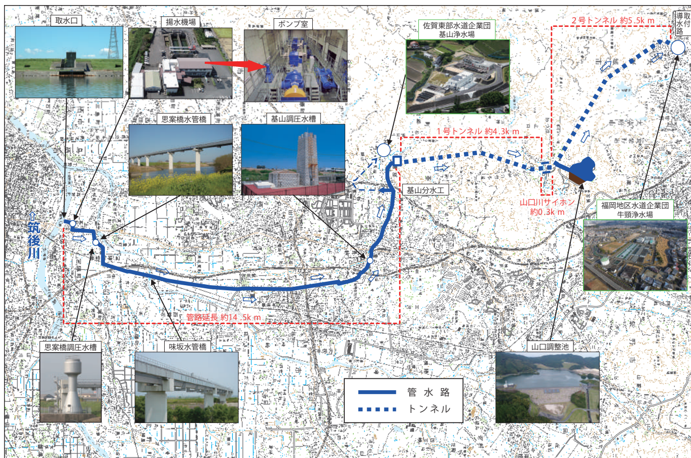
福岡導水縦断面図
