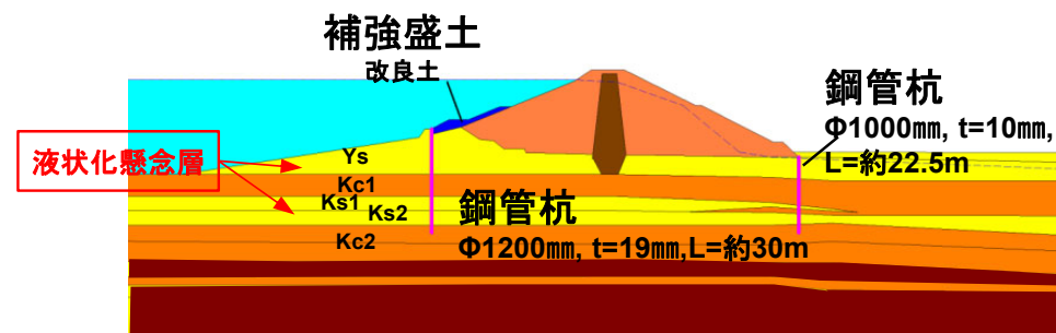
標準断面図
