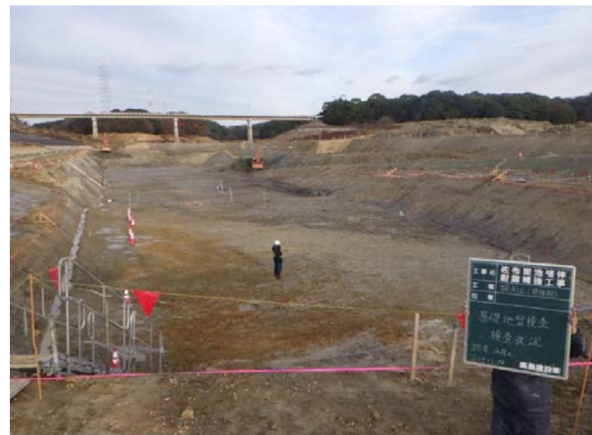
堤体掘削完了
