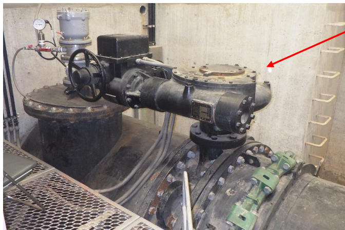
別図（大別れ制水弁 現況写真）
