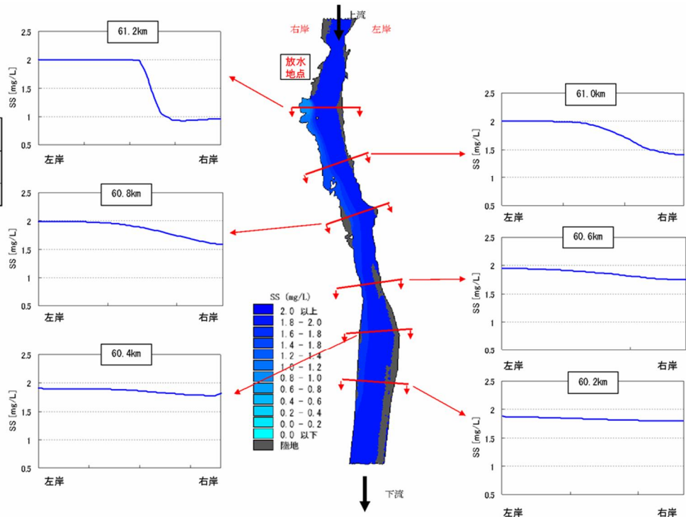
木曾川 SS 予測結果(局所的な混合(異常湧水時)・61.2km 付近に放水)
