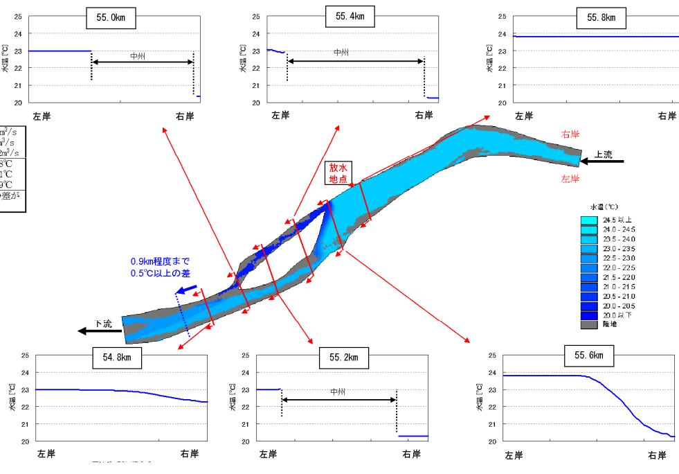
長良川 水溫予測結果(局所的な混合(異常渇水時)・55.6km 付近に放水)
