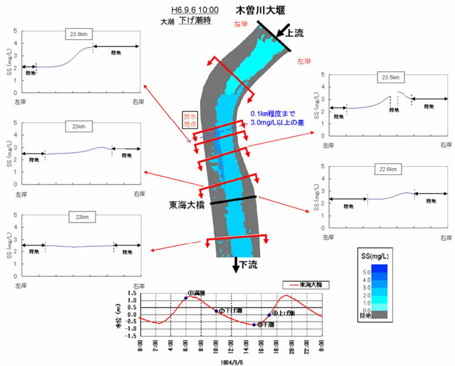
木曾川 SS 予測結果(局所的な混合(異常湧水時)・24.0km 付近に放水)
