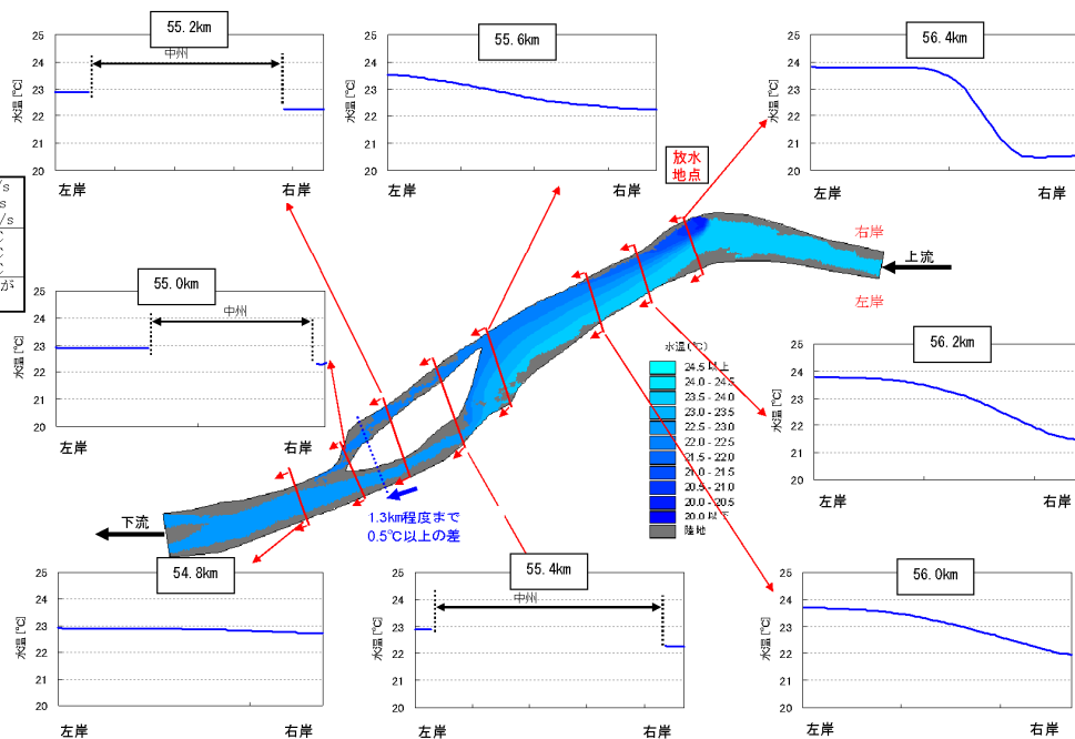
長良川 水溫予測結果(局所的な混合(異常渇水時)・56.4km 付近に放水)
