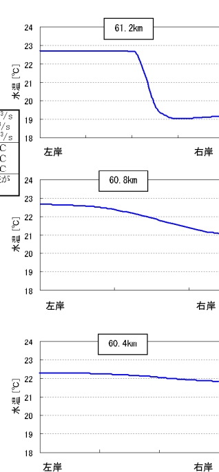
木曾川 水温予測結果(局所的な混合(異常温水時)・61.2km 付近に放水)
