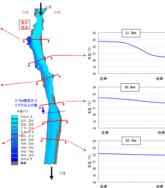
木曾川 水温予測結果(局所的な混合(異常温水時)・61.2km 付近に放水)
