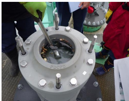
空気弁の分解
