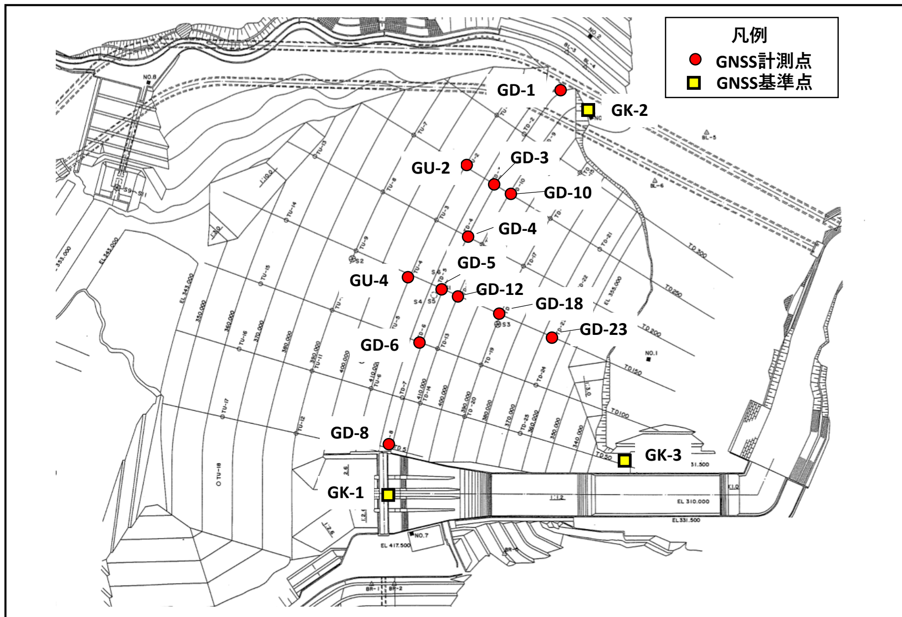
GNSS計測点及び基準点配置図（阿木川ダム）
