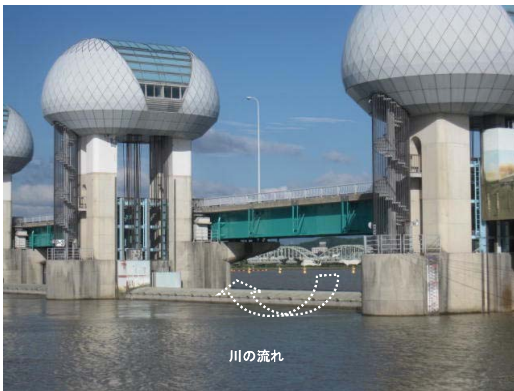
ゲート全開操作終了後の長良川河口堰（アンダーフロー操作に切り替え） 8月9日 7時撮影
