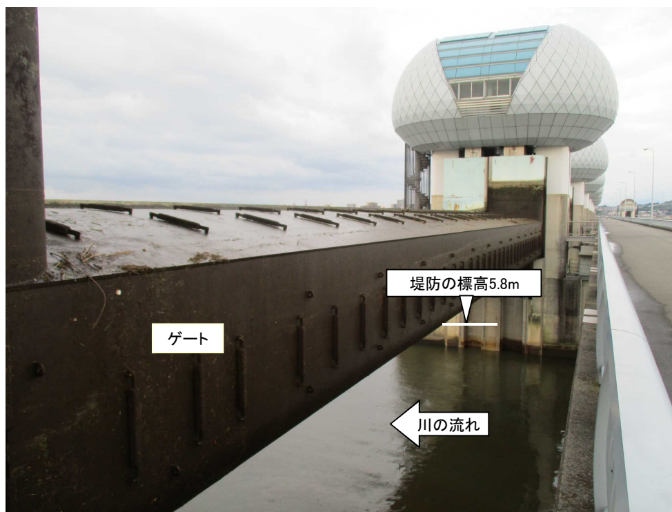
ゲート全開操作開始後の長良川河口堰（堤防より高い位置にゲートを引き上げ） （2回目）
