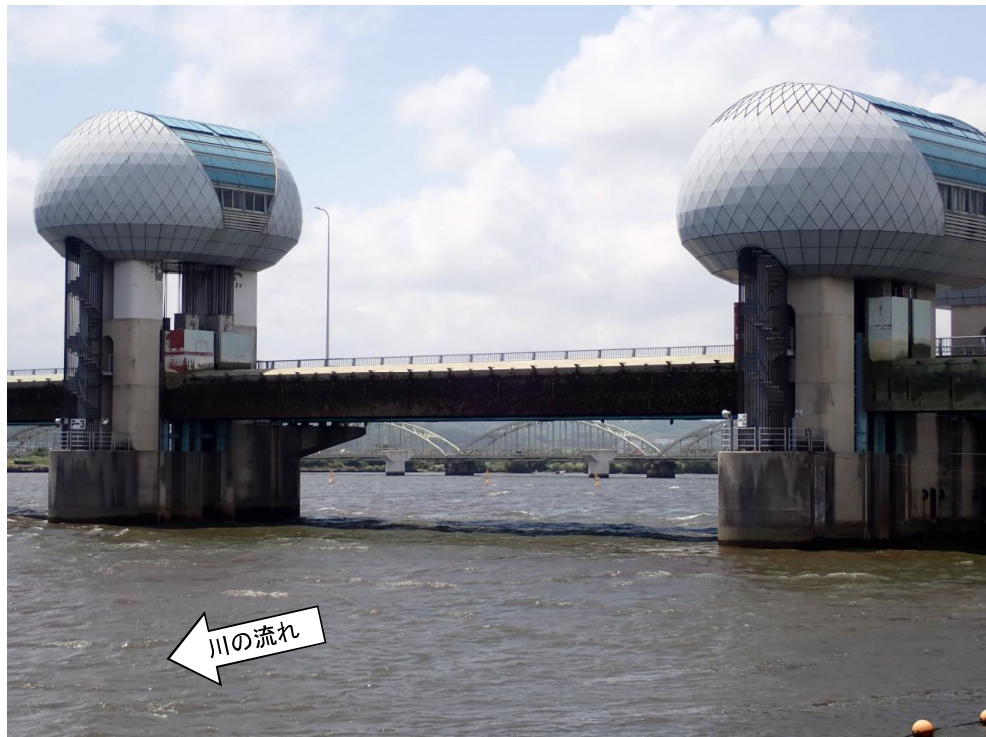
堰下流側
