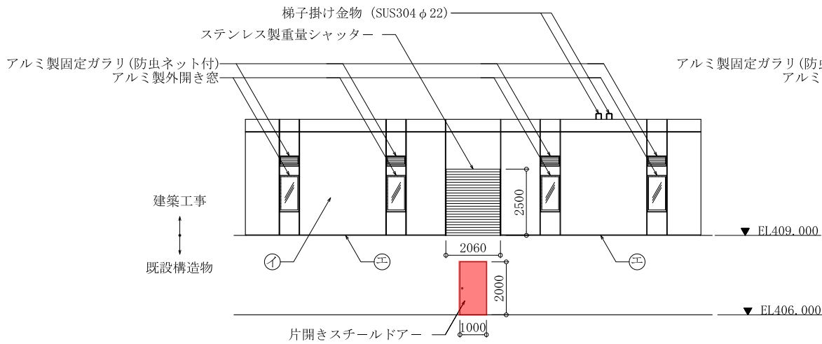
下流面
