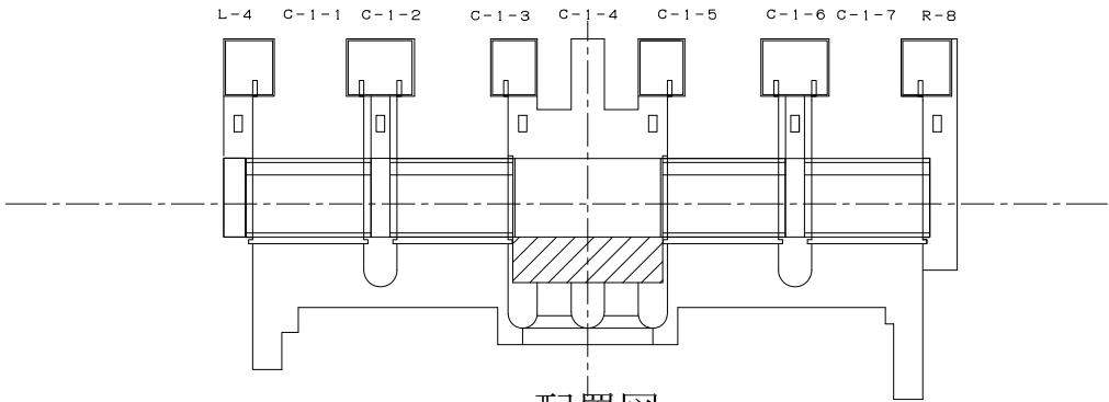
配置図
