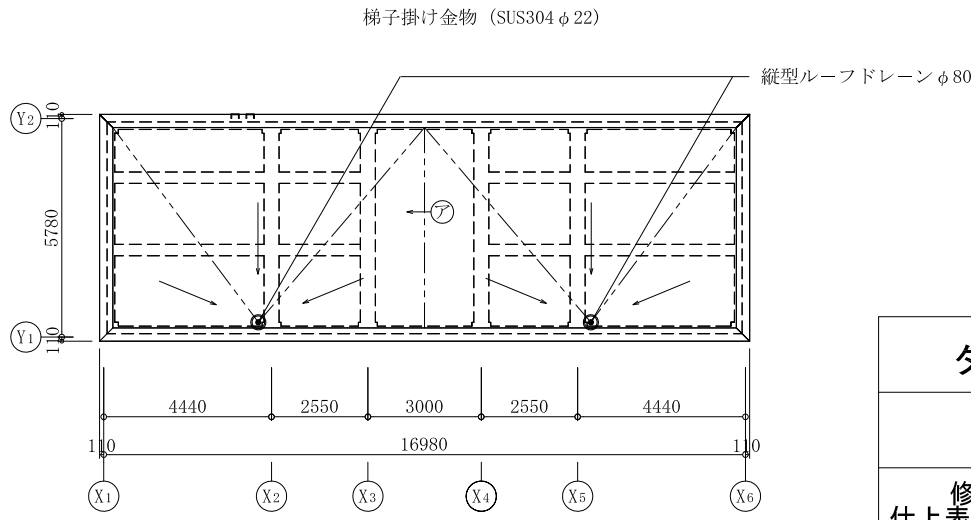
屋根伏図
