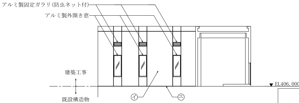
常用洪水吐側
