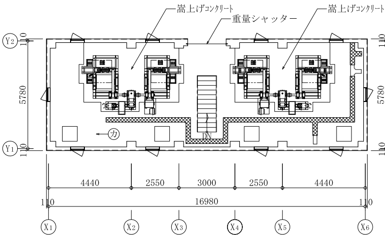
1階平面図
