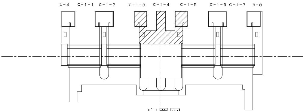
配置図
