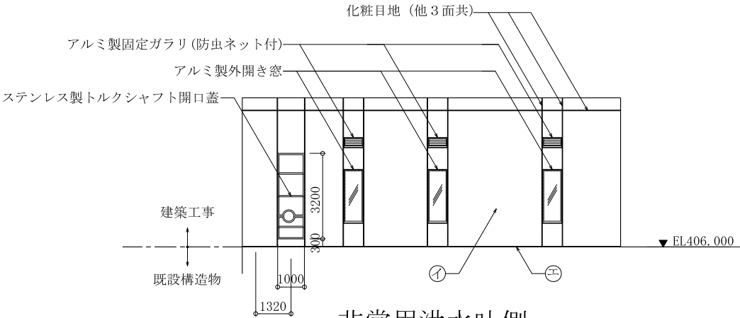
非常用洪水吐側
