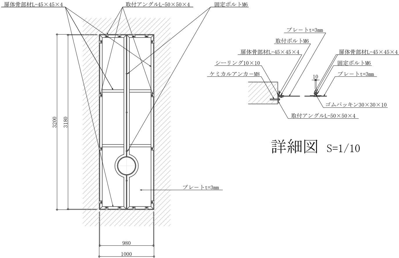
トルクシャフト開口部蓋 S=1/20
