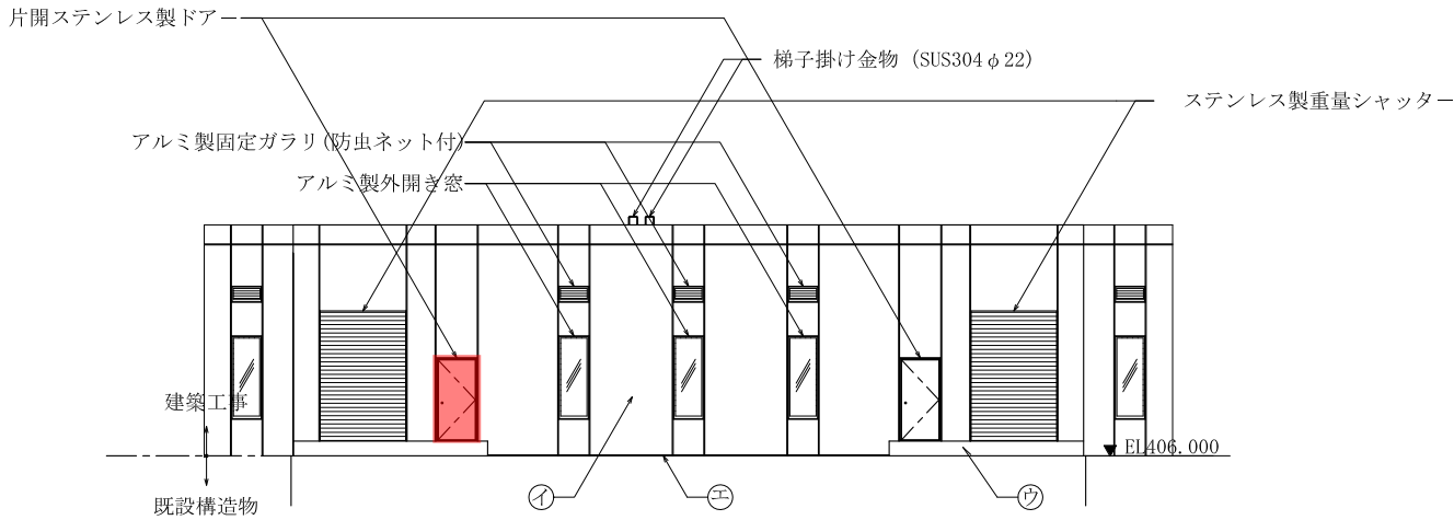
上流面
