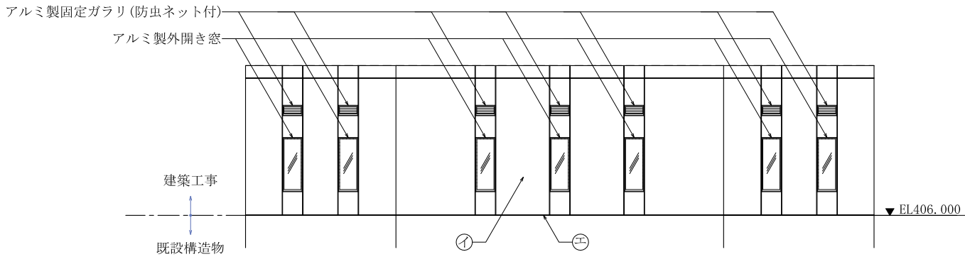
下流面
