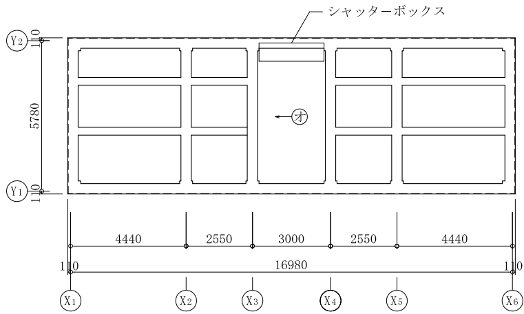
天井伏図
