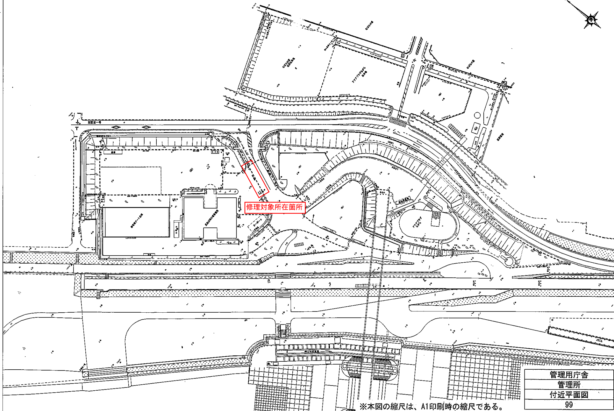
付 近 平 面 図 S=1/500
