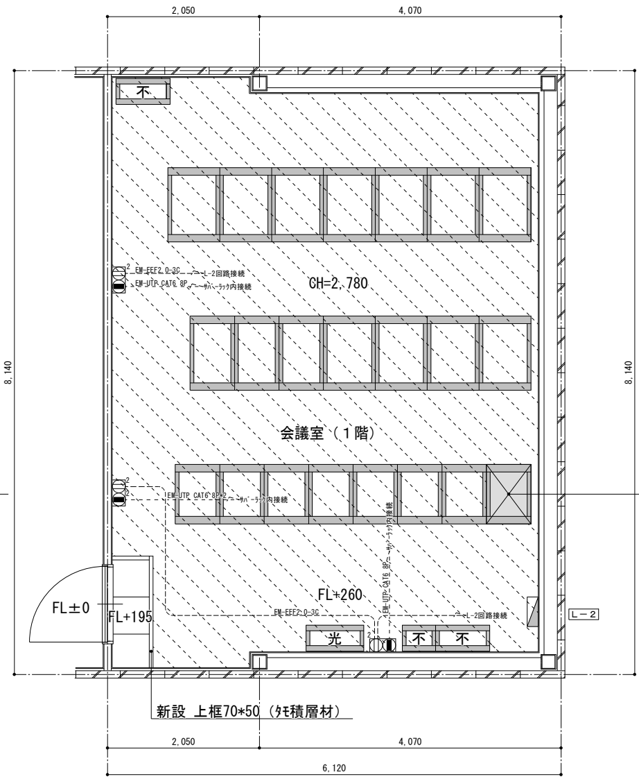
整備平面詳細図 S=1/50
