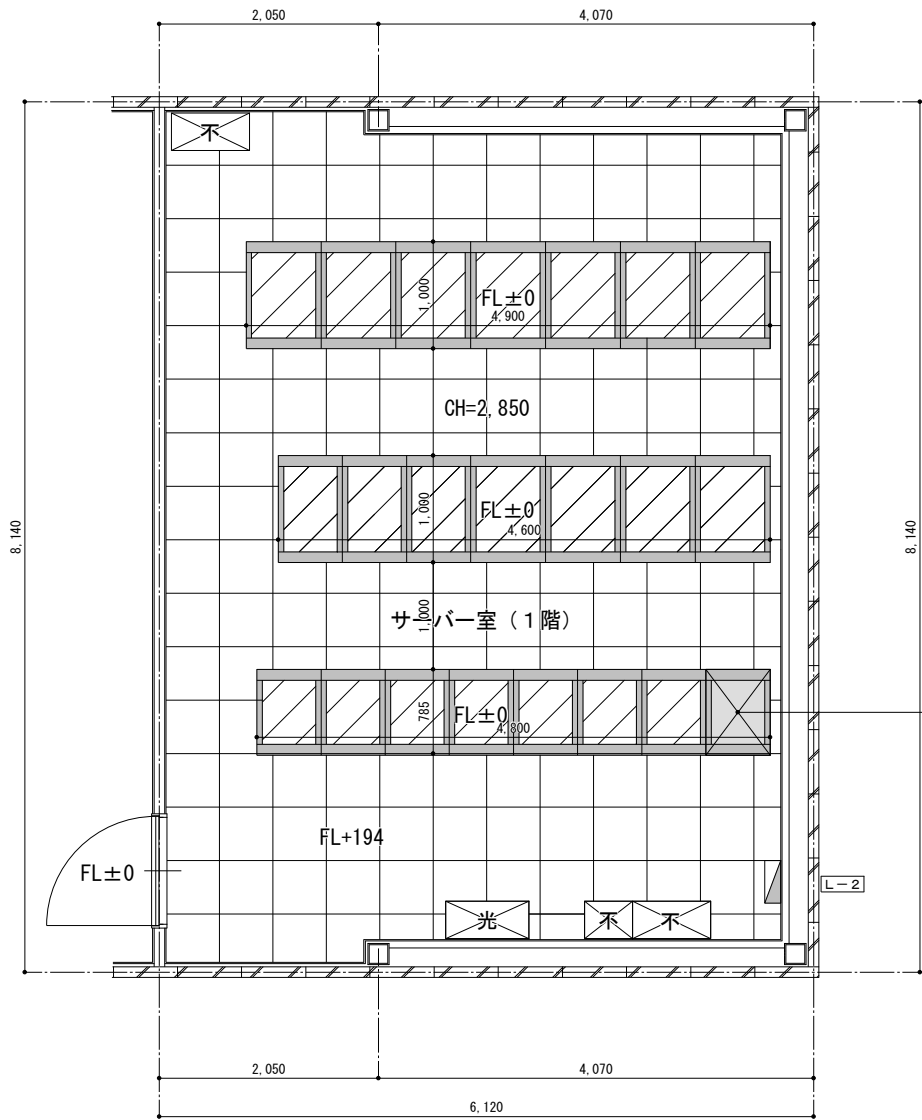
現況平面詳細図 S=1/50
