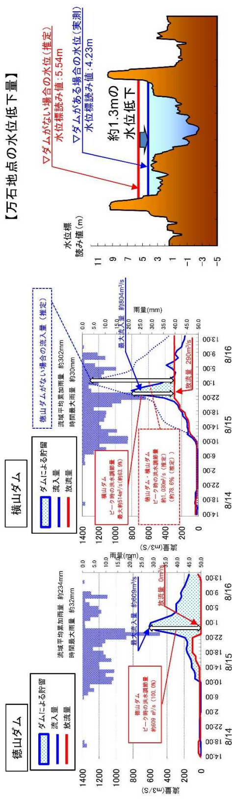
【徳山ダム・横山ダム連携による洪水調節】
