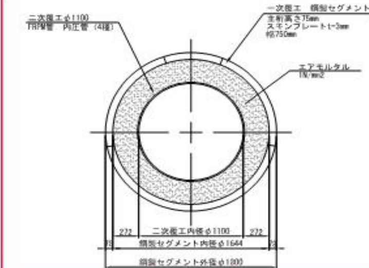
幹線水路・併設水路(シールド)標準断面図
