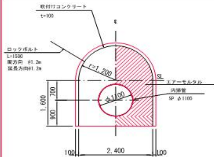
幹線水路・併設水路(トンネル)標準断面図
