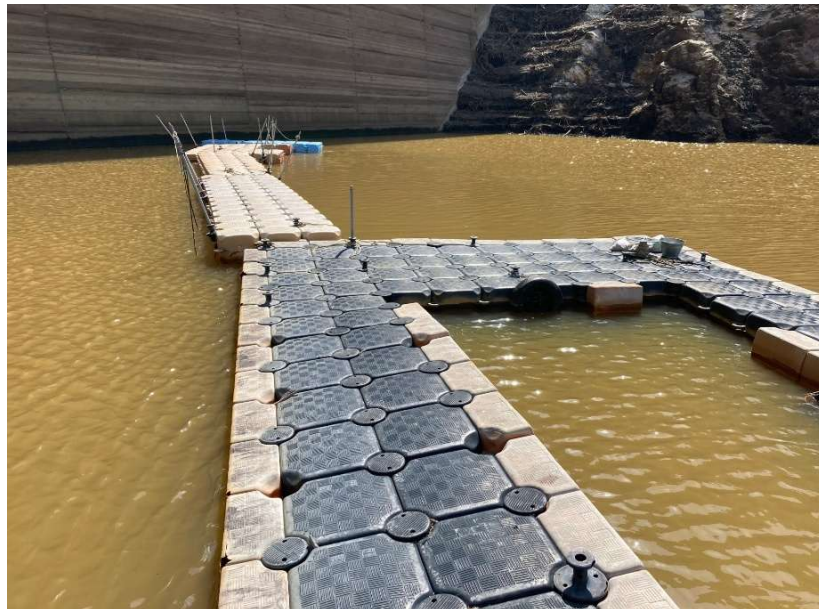
<浮棧橋設置> (既設・宇連)
