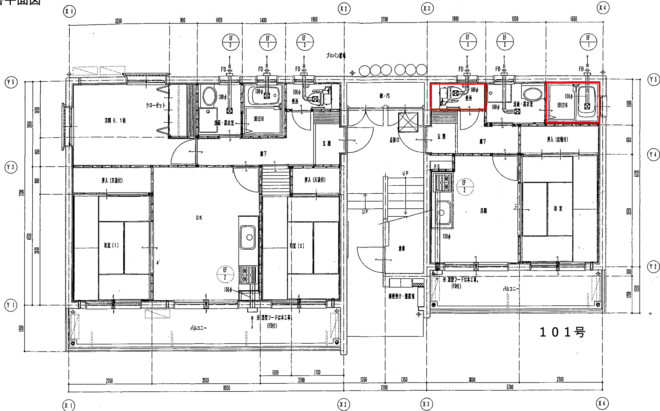
Aタイプ 1~2階平面図 S=1/50
