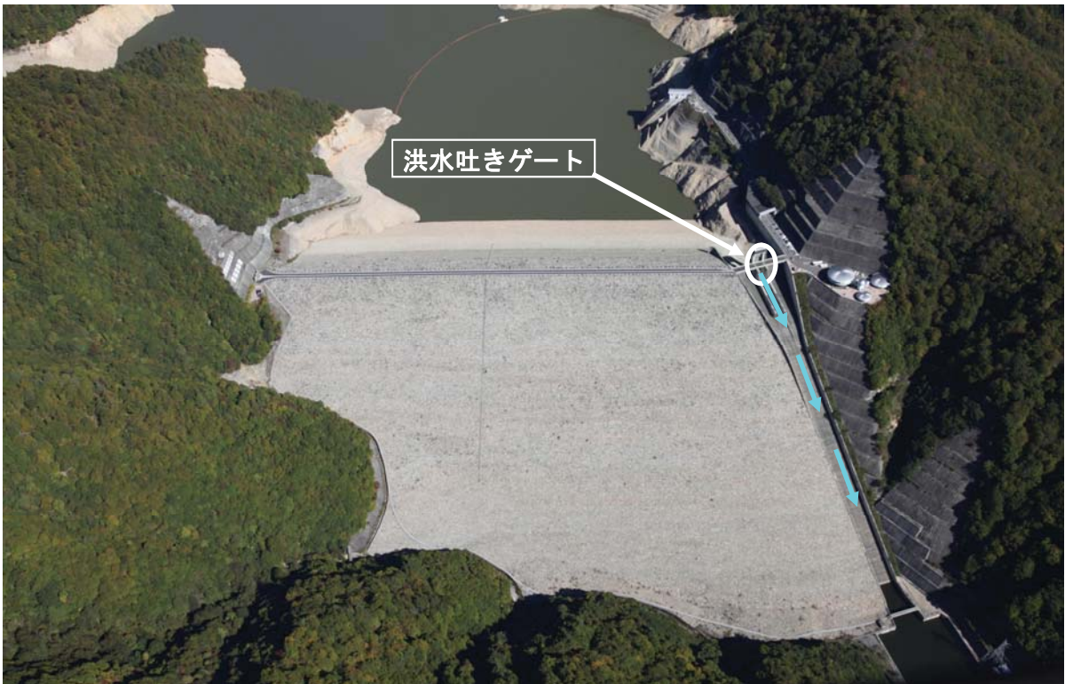
奈良俣ダム洪水吐きゲート
