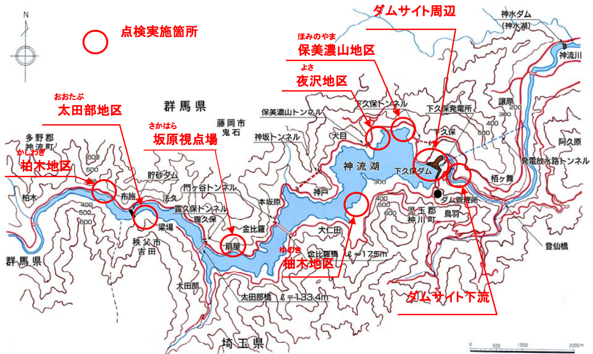
下久保ダム及び神流湖周辺平面図
